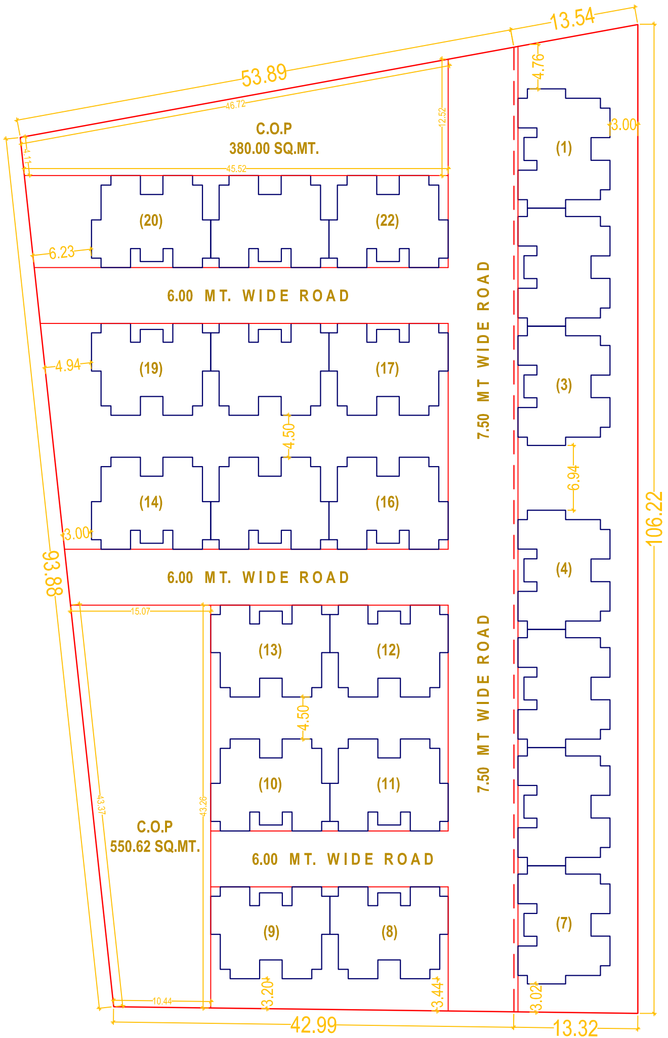
LAY OUT PLAN FOR T.P.47(Bhestan), F.P.No. R-10
